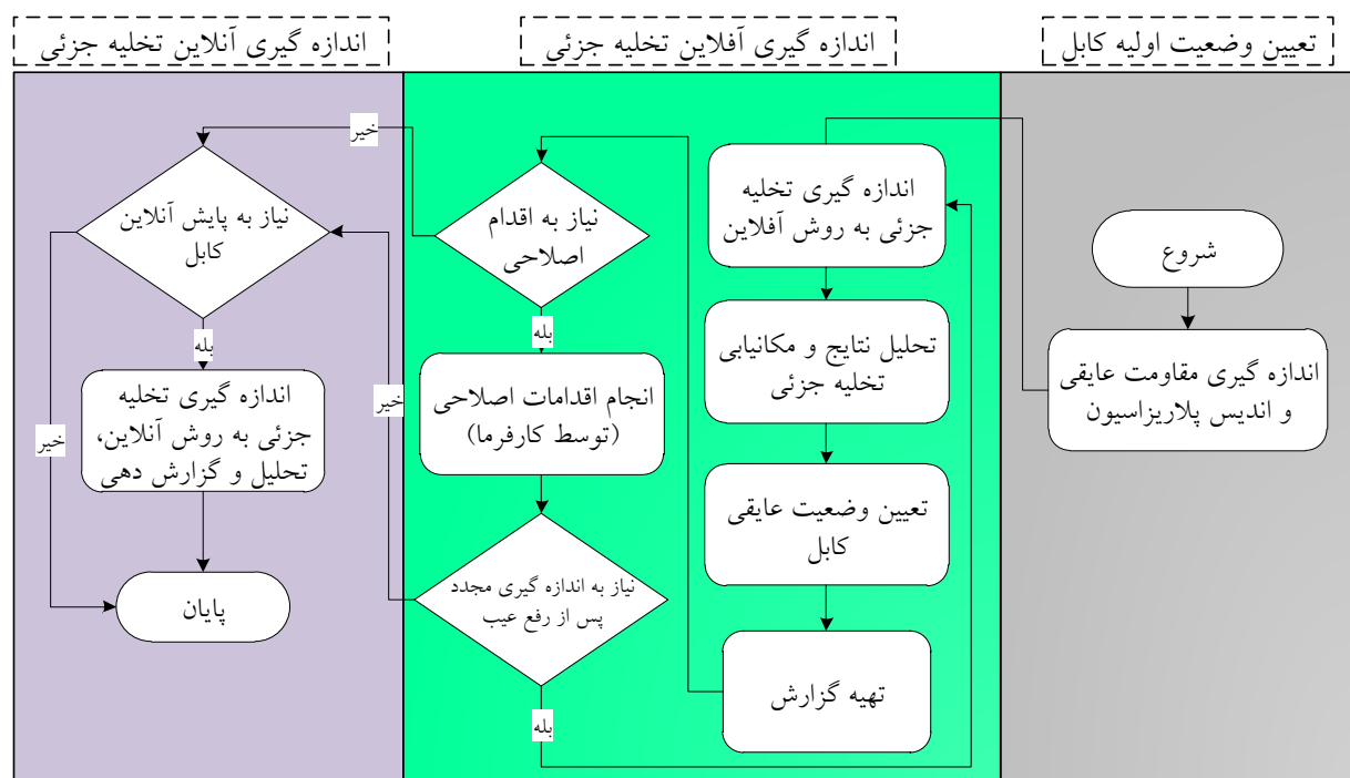
شکل ۱: فلوجارت نحوه انجام آزمون کابل‌های تحت پیمان
